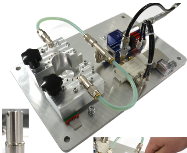
Ręczny system olejowy do uszczelnienia wargowego.
