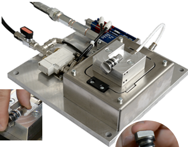
Ręczny system smarowania części gumowych.
