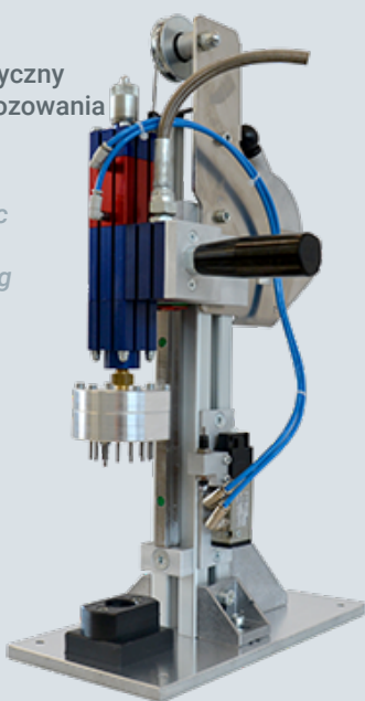
Ręczny wolumetryczny system smarowania na przekładni.
