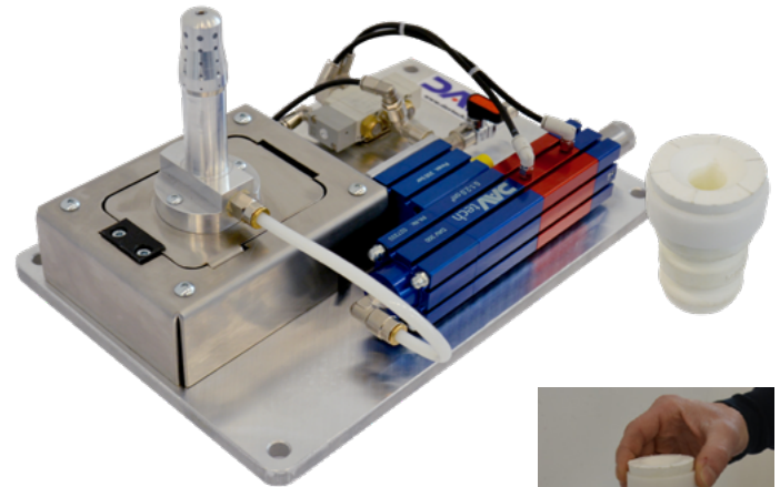
Ręczny system smarowania części gumowych.
